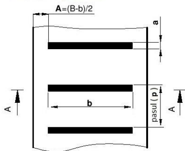
1. Banda transportoare cu racleti transversali pe un rand
