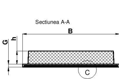
1. Banda transportoare cu racleti transversali pe un rand
