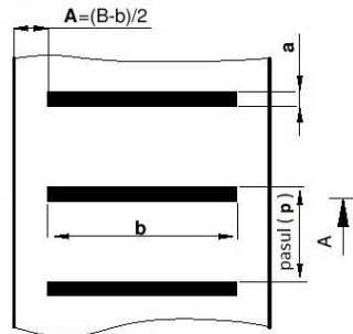
1. Banda transportoare cu racleti transversali pe un rand
