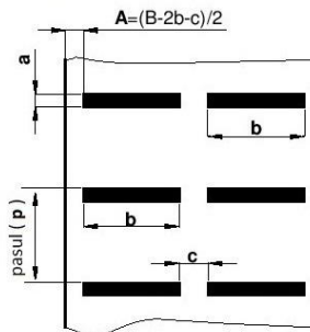
2. Banda transportoare cu racleti transversali pe doua randuri
