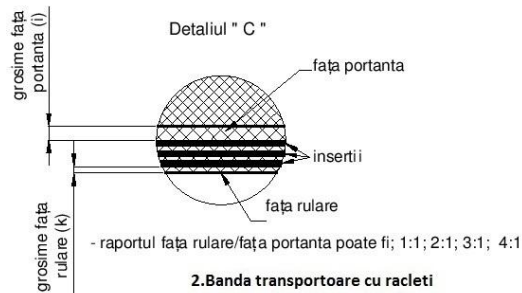
2. Banda transportoare cu racleti transversali pe doua randuri
