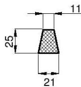
Profil racleti
