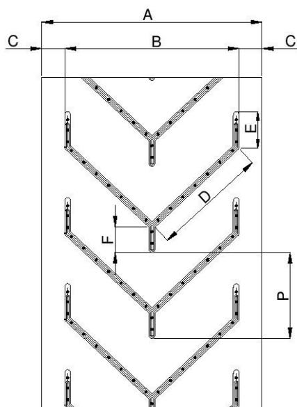
Profil racleti
