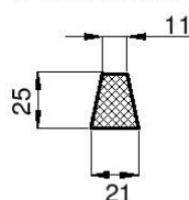
Profil racleti
